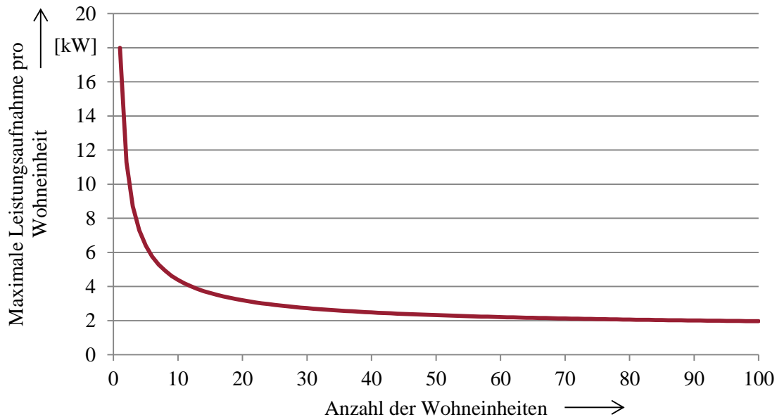
Abbildung 15-2: Maximale gleichzeitige Leistungsaufnahme pro Wohneinheit
