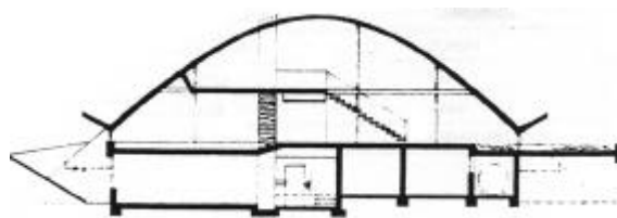
Abb. 4.2.14: Wohnhaus X1, Schnitt Q: Baumeister, 1964, S. 1408-1413
