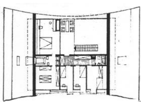
Abb. 4.2.16: Wohnhaus X1, Obergeschoß Q: Baumeister, 1964, Jg. 61, S. 1408-1413
