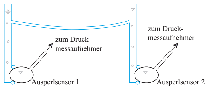
Bild 4.7: Prinzipskizze einer verbesserten Kalibriervorrichtung (blau)
