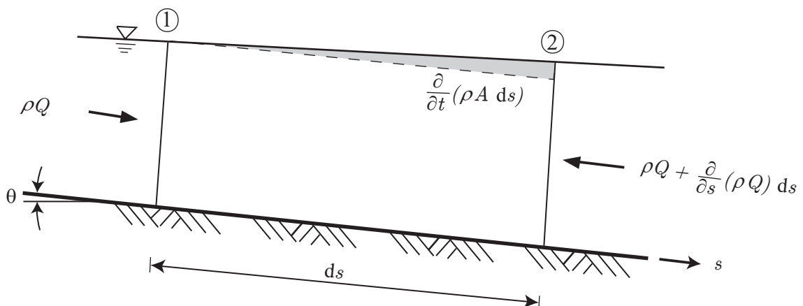
Bild 3.2: Massenerhalt im Kontrollraum (eindimensional, instationär)
