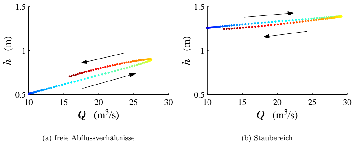
Bild 7.15: Hysterese zwischen der Wassertiefe und dem Durchfluss
