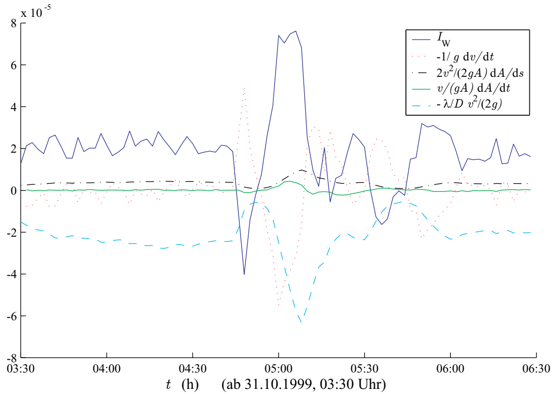
Bild 7.20: Einfluss der Terme bei instationärer Berechnung für sehr schnelle Durchflussänderungen
