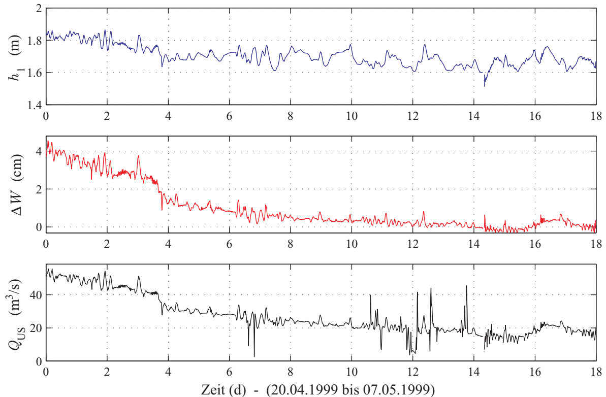
Bild 5.2: Messwerte für einen Zeitabschnitt mit groben Fehlern (ohne Korrektur)
