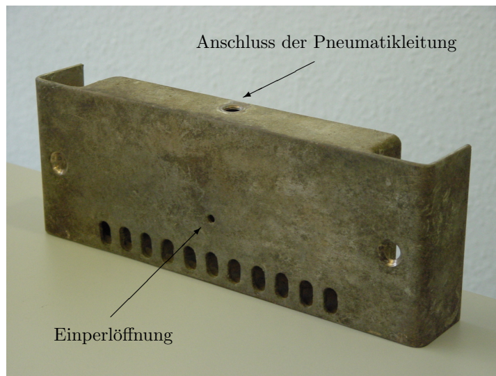
Bild 4.5: Erster am Pegel Fröndenberg montierter Einperlsensor aus Metall (Fa. Ott Hydrometrie, 1998)
