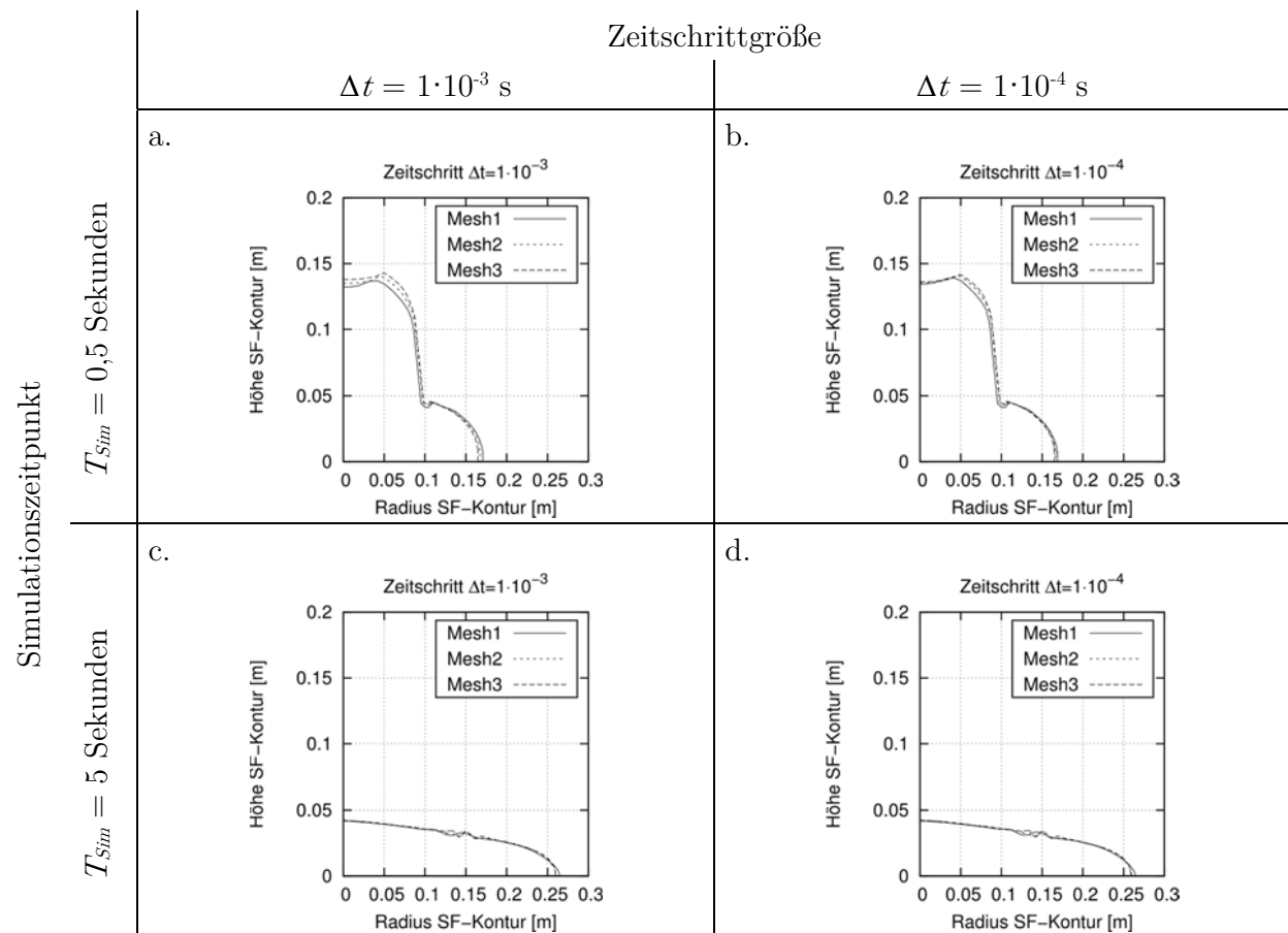
Bild 33 Vergleich der Setzfließmaßkonturen für die Simulationszeitpunkt T_{Sim} = 0,5 \text{ Sekunden} und T_{Sim} = 5 \text{ Sekunden} für die Zeitschrittgrößen \Delta t = 1 \cdot 10^{-3} \text{ s} und \Delta t = 1 \cdot 10^{-4} \text{ s}
