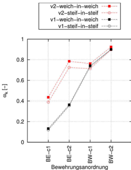
Bild 87 Ergebnis der Auswertung der Untersuchungsparameter auf das Flächenverhältnis \alpha_K getrennt dargestellt für die Kombinationen mit gleichen (a.) und unterschiedlichen (b.) Fluidparameter-sätzen
