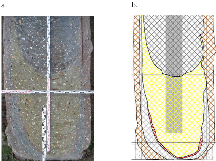
Bild 75 Foto (a.) mit kolorierte Skizze (b.) des Längsschnittes im Bereich des Pfahlfußes des unter Flüssigkeitsstützung hergestellten Probepfahls mit Bewehrungskorb [15]
