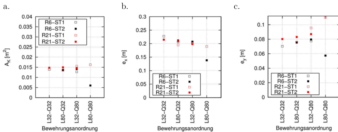
Bild 53 A_K (a.), e_x (b.) und e_y (c.) in Abhängigkeit der Versuchsparameter für den Querschnitt 2 bei z = 0,4 \text{ m}
