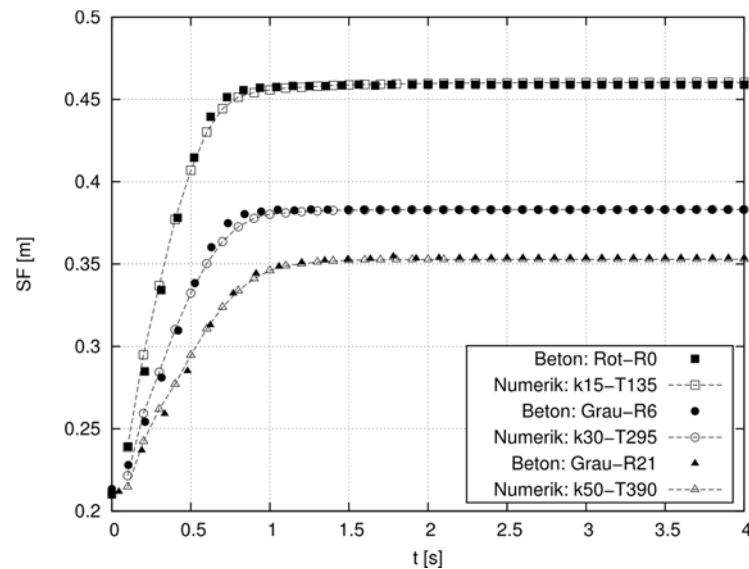
Bild 56 Vergleich der Ergebnisse der zeitabhängigen Setzfließmaße SF aus den Laborversuchen mit den Ergebnissen aus den zugehörigen numerischen Simulationen, die jeweils die beste Übereinstimmung liefern
