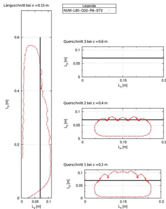
Bild 58 Darstellung der Kontur des einströmenden Fluides 2 im Längsschnitt und in den Querschnitten als Ergebnis der numerischen Simulation der Versuchskombination L32-Q80-R6-ST2 für den letzten Simulationszeitpunkt ( T_{Sim} = 2,5 s)
