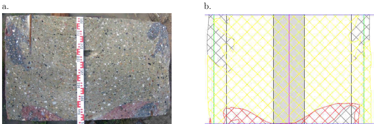
Bild 6 Foto (a.) und kolorierte Skizze (b.) des Längsschnittes des verrohrt hergestellten Probepfahls mit Bewehrungskorb [15]
