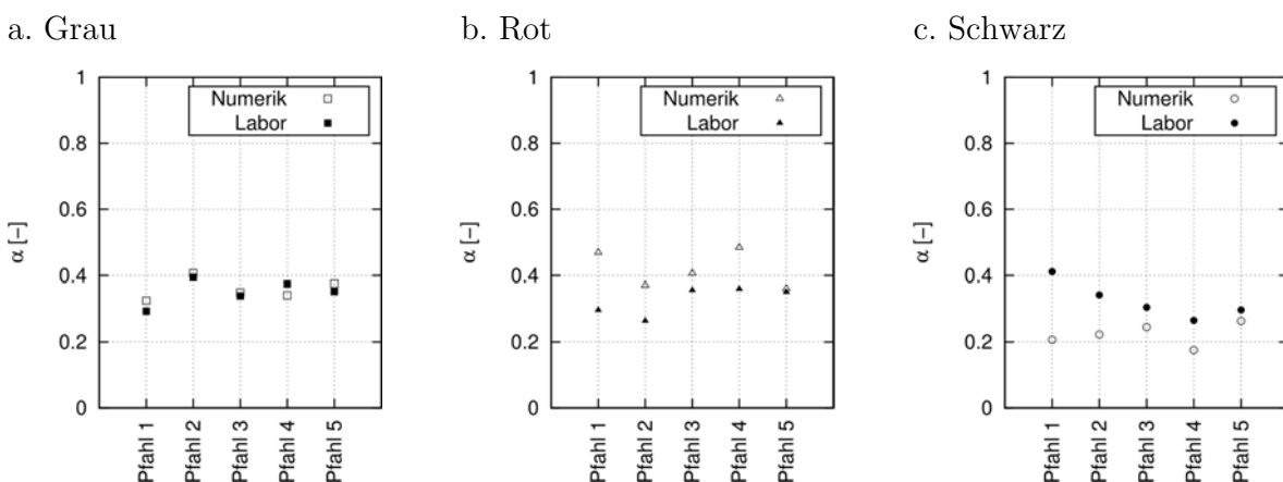
Bild 71 Auswertung des Flächenverhältnis \alpha im Längsschnitt für die graue (a.), rote (b.) und (c.) schwarze Charge
