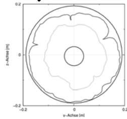
Bild 104 Ergebnis des Laborversuches: Konturdaten des Modellpfahls P4
