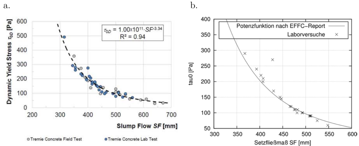
Bild 44 (a.) Beziehung zwischen dem Setzfließmaß und der Fließgrenze nach [38]; (b.) Beziehung zwischen der Setzfließmaß und dem Fließgrenzenparameter \tau_{00} dieser Arbeit mit Darstellung der gefitteten Potenzfunktion nach [38]
