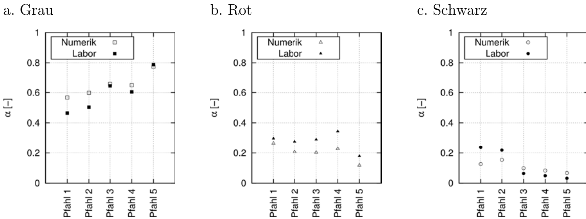
Bild 69 Auswertung des Flächenverhältnis \alpha im Querschnitt 1 für die graue (a.), rote (b.) und (c.) schwarze Charge
