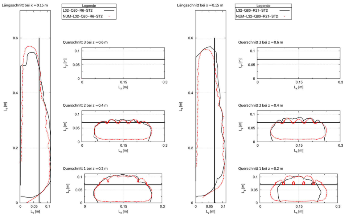
Bild 59 Vergleich der Kontur der roten Frischbetoncharge des physikalischen Versuches mit der zugehörigen numerischen Simulation für die Versuchskombinationen L32-Q80-R6-ST2 (a.) und L32-Q80-R21-ST2 (b.)
