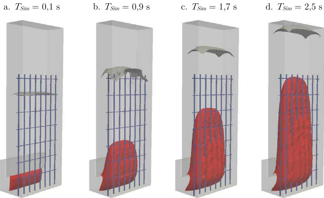
Bild 57 Darstellung der Kontur des einströmenden Fluides als Ergebnis der numerischen Simulation der Versuchskombination L32-Q80-R6-ST2 für die Simulationszeitpunkte T_{Sim} = 0,1 s (a.), T_{Sim} = 0,9 s (b.), T_{Sim} = 1,7 s (c.) und T_{Sim} = 2,5 s (d.)
