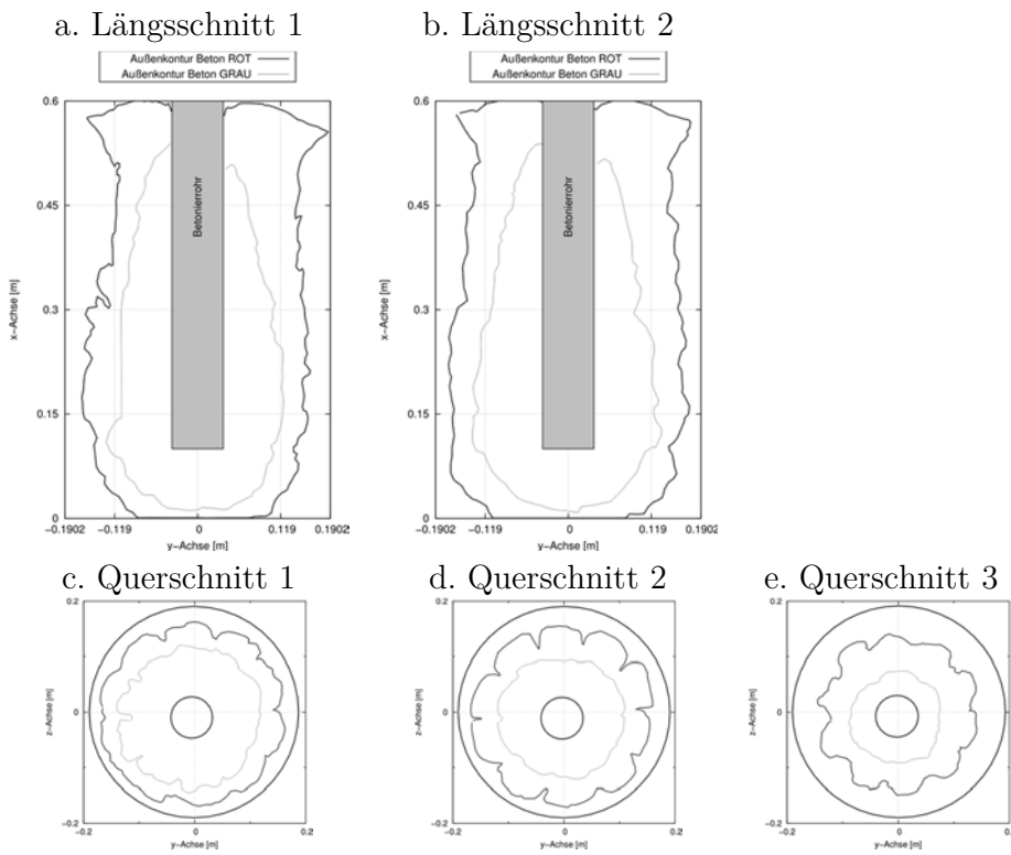
Bild 101 Ergebnis des Laborversuches: Konturdaten des Modellpfahls P1
