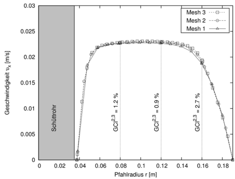
Bild 106 Geschwindigkeitsprofil über den Pfahlradius r bei h = 0,5 m für Mesh1, Mesh2 und Mesh3 mit Angabe des GCI^{2,3}_{fine} an ausgewählten Koordinaten
