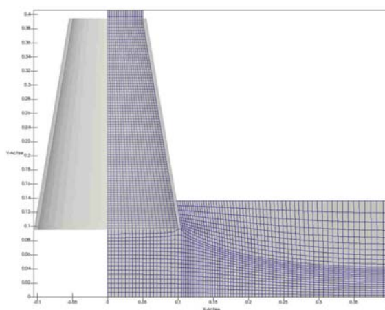
Bild 32 Dreidimensionale Darstellung (a. und b.) und Ansicht (b. und c.) des numerischen Modells mit Darstellung des Berechnungsnetzes für den Setzfließmaßversuch vor und nach Ziehen des Prüfkonus
