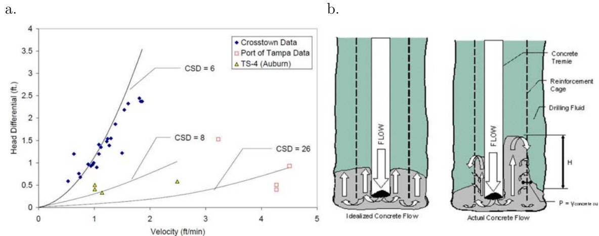
Bild 5 (a.) Beziehung zwischen der Steiggeschwindigkeit und des Pegelunterschiedes innerhalb und außerhalb des Bewehrungskorbes [13]; (b.) Idealisierte (links) und tatsächliche Strömungsvorgänge (rechts) des Frischbetons in einem Bohrpfahl [13]
