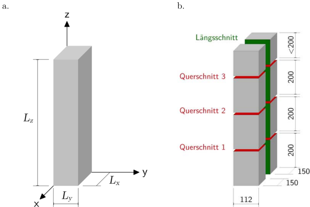
Bild 48 Schematische Skizzen des ausgeschalteten Betonblockes: (a.) Definition der Achsen und Bezeichnung der Abmessungen; (b.) Schnittbezeichnung und Abmessungen in [mm]
