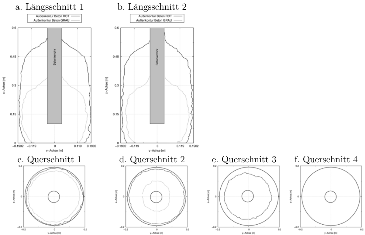
Bild 105 Ergebnis des Laborversuches: Konturdaten des Modellpfehls P5
