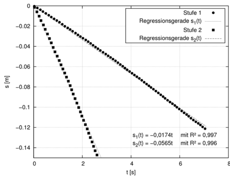
Bild 96 Weg-Zeit-Messung des Absenkvorganges des Laborkranses für zwei Geschwindigkeitsstufen
