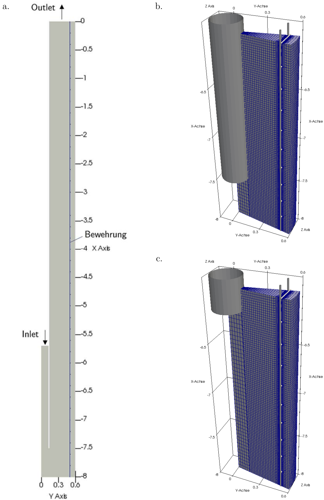
Bild 78 (a.) Ansicht des Keilmodelles mit den Abmessungen in [m]; Dreidimensionale Detailausschnitte des Berechnungsgitters am Pfahlfuß mit Darstellung des Kontraktorrohres für den Ausgangszustand (b.) und nach Ziehen des Kontraktorrohres (c.)
