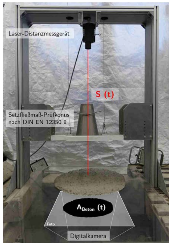
Bild 26 Bearbeitetes Foto des modifizierten Setzfließmaßversuchsstandes
