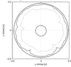
Bild 103 Ergebnis des Laborversuches: Konturdaten des Modellpfahls P3
