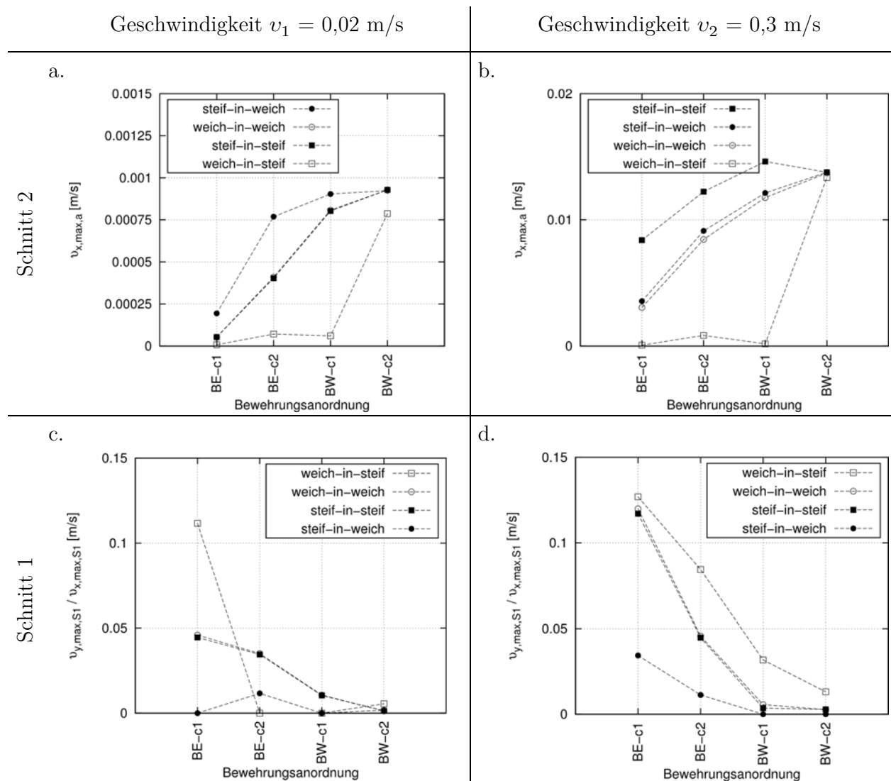
Bild 90 Absolute Geschwindigkeit v_{x,max,a} im Schnitt 2 (a. und b.) und das Geschwindigkeitsverhältnis v_{y,max} / v_{x,max} im Schnitt 1 (c. und d.) für T_{Sim} = 34 min und beide Einströmgeschwindigkeiten
