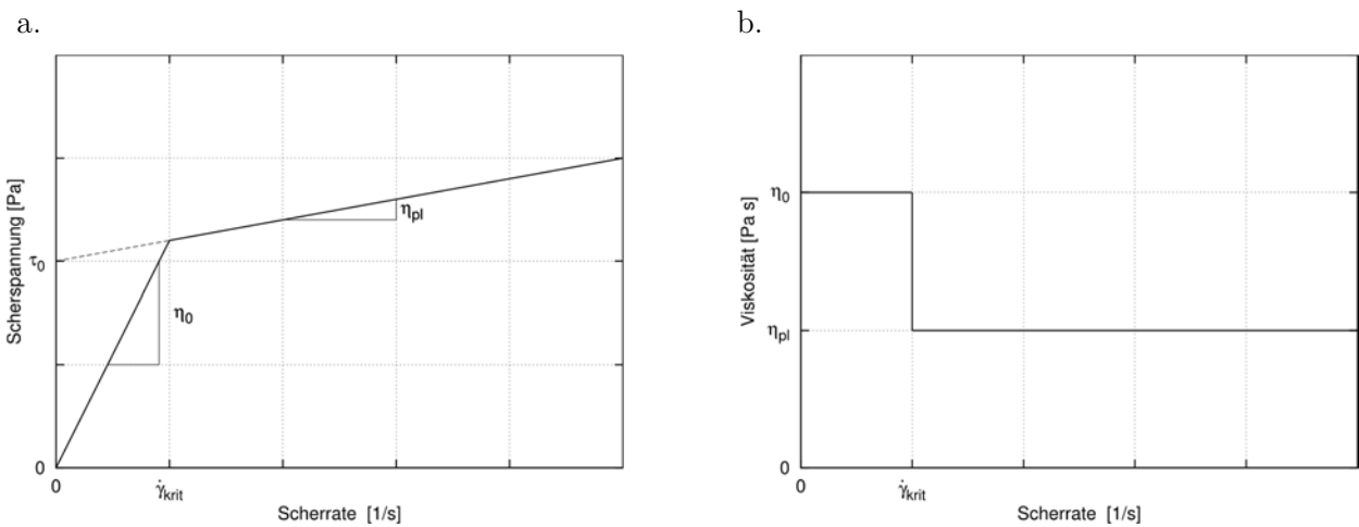
Bild 18 Scherraten-Scherspannungs-Beziehung (a.) und Scherraten-Viskositäts-Beziehung (b.) des Bi-Viskositätsmodelles für das in OpenFOAM implementierte Herschel-Bulkley-Modell mit n = 1
