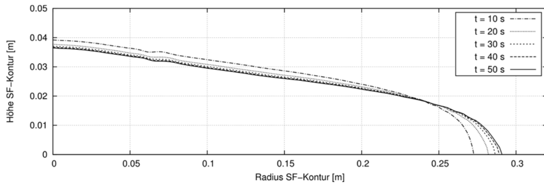
Bild 24 Vergleich der Setzfließmaßkontur für das Mesh2 und einen Zeitschritt von \Delta t = 1 \cdot 10^4 s für unterschiedliche Zeitpunkte während des Ausbreitprozesses für den „virtuellen“ Frischbeton ( \tau_0 = 50 Pa, \eta_{Pl} = 50 Pa \cdot s, \rho = 2.300 kg/m 3 )
