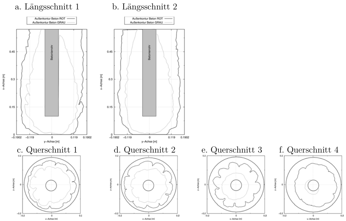
Bild 102 Ergebnis des Laborversuches: Konturdaten des Modellpfahls P2
