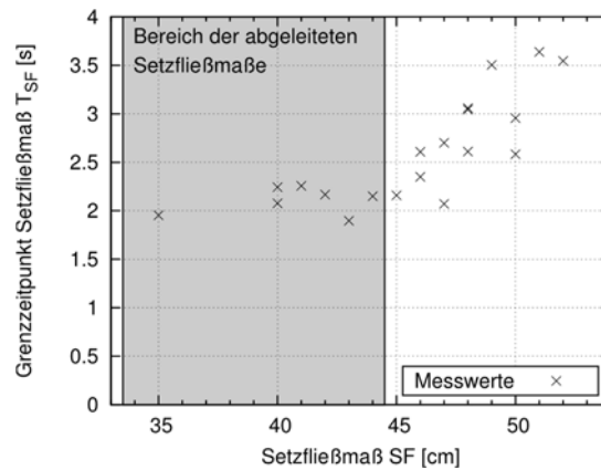
Bild 82 Abhängigkeit zwischen dem Setzfließmaß SF und dem Grenzzeitpunkt T_{SF} für die in den eigenen Laborversuchen untersuchten Mischungsentwürfe
