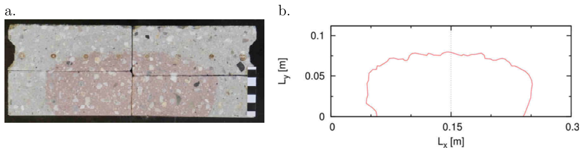
Bild 49 Gegenüberstellung des originalen Fotos (a.) mit der digital erzeugten Kontur (b.) des roten Betons für den Querschnitt 2 bei z = 0,4 \text{ m} (L32-Q80-R6-ST2)
