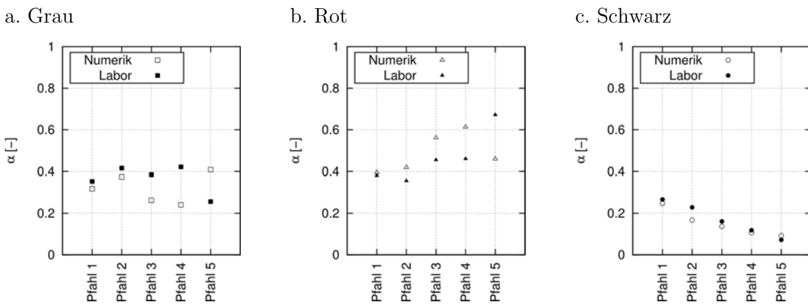
Bild 70 Auswertung des Flächenverhältnis \alpha im Querschnitt 2 für die graue (a.), rote (b.) und (c.) schwarze Charge
