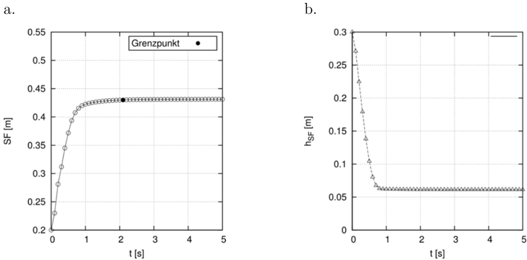
Bild 38 Zeitabhängiges Setzfließmaß SF (a.) und die Höhe h_{SF} des Kegelstumpfes in Achsmittle (b.) als Ergebnis der numerischen Simulation mit \tau_{u0} = 170 \text{ Pa} , k = 22 \text{ Pa}\cdot\text{s} und \rho = 2300 \text{ kg/m}^3
