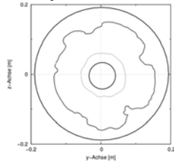
Bild 103 Ergebnis des Laborversuches: Konturdaten des Modellpfahls P3
