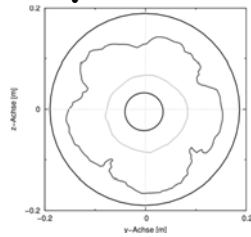
Bild 104 Ergebnis des Laborversuches: Konturdaten des Modellpfahls P4
