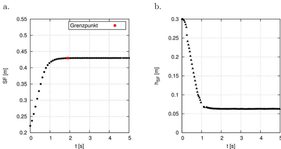
Bild 29 Zeitabhängiges Setzfließmaß SF (a.) und zeitabhängige Höhe h_{SF} des Kegelstumpfes in Achsmittelle (b.) als Ergebnis des physikalischen Versuches RB16-FM025-0
